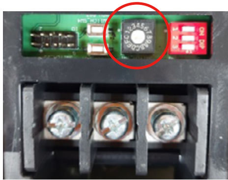
輸出電流調整開關
